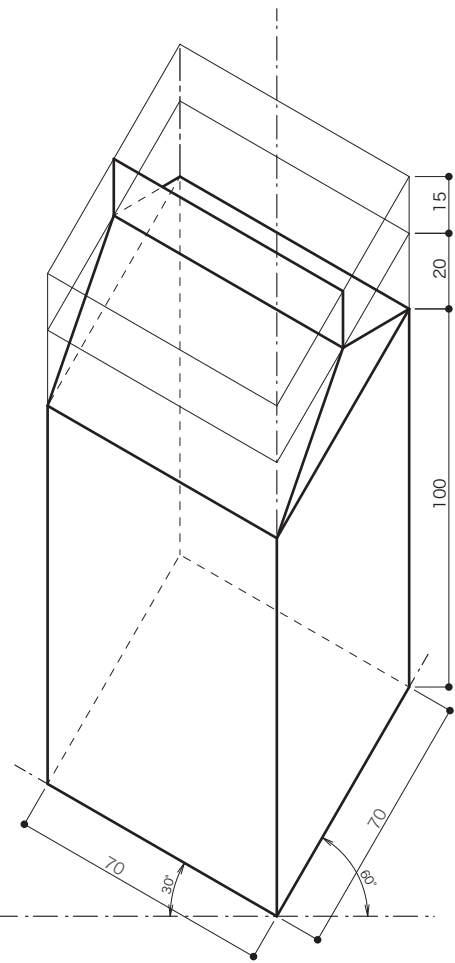
アクソメトリック図(30°-60°) S=1:2
