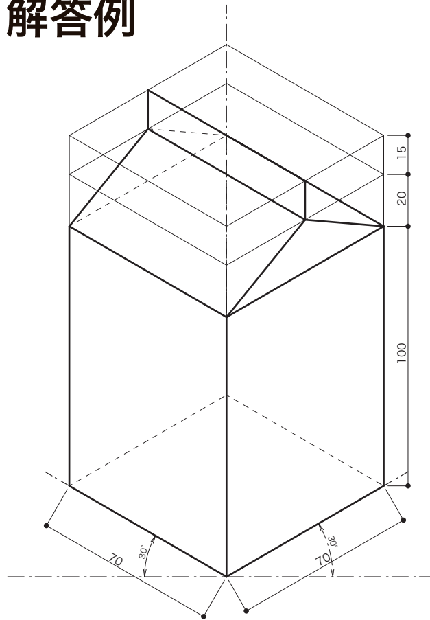
アイソメトリック図 S=1:2
