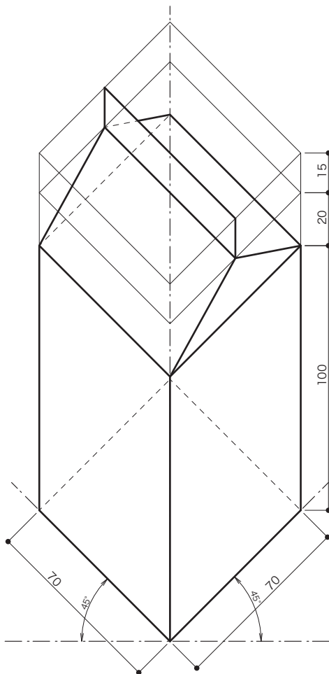
アクソメトリック図(45°-45°) S=1:2
