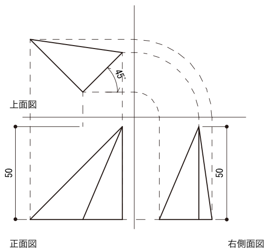
立体C：三角錐 S=1:2
