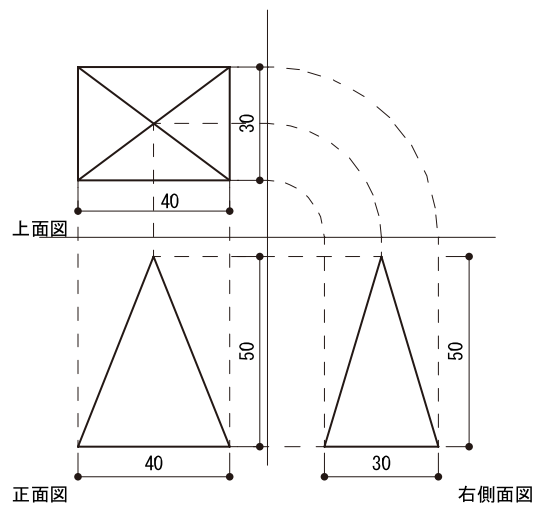
立体B：四角錐 S=1:2
