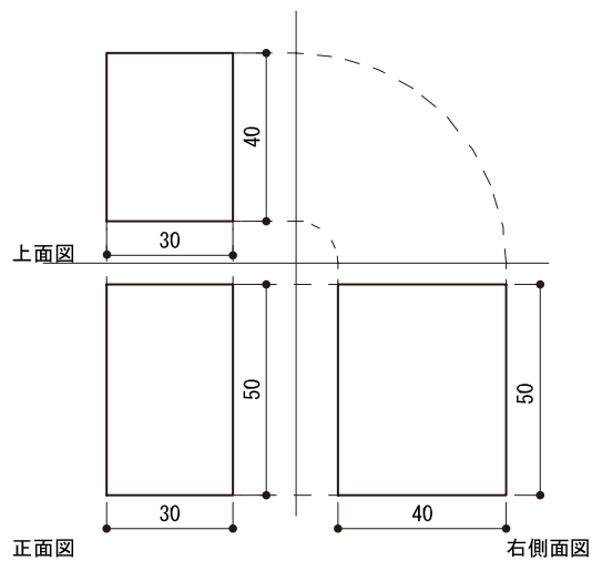
立体A：直方体 S=1:2
